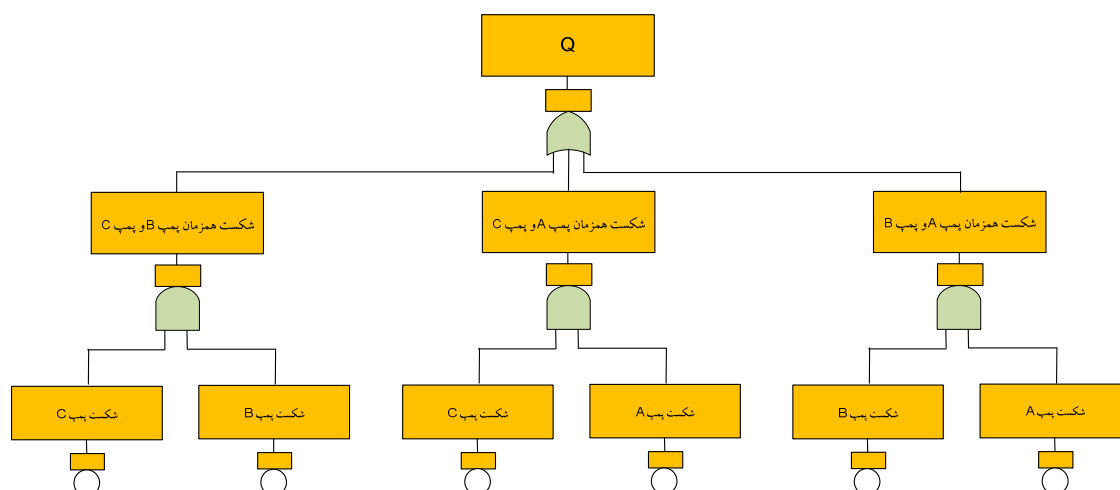
تصویر ۸-۴: درخت خطای مربوط به توقف عملیات انتقال گاز
