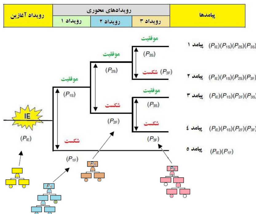
تصویر ۲-۵: کمی نمودن درخت واقعه
