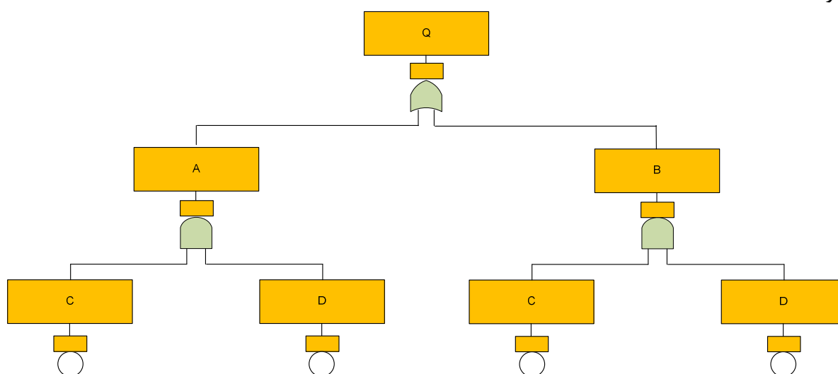
تصویر ۶-۸: درخت خطای معادل تصویر ۶-۷
