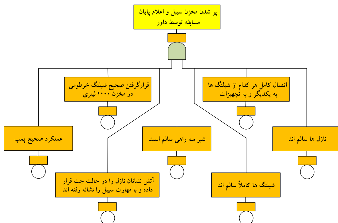
تصویر د-۲: درخت موفقیت مسابقه آبرسانی
