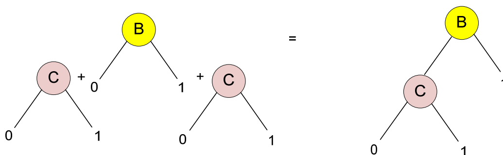
تصویر ۱۱-۶: اجرای تابع OR با استفاده از روش BDD (مرحله ۲)
