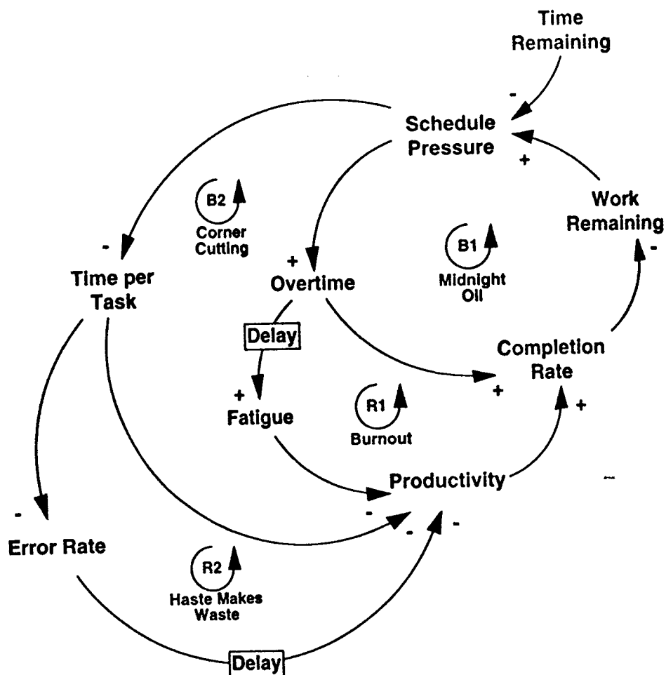
شکل ۸-۵: شماره گذاری و نام گذاری حلقه‌های بازخوردی اصلی برای شفاف شدن و درک بهتر مدل
