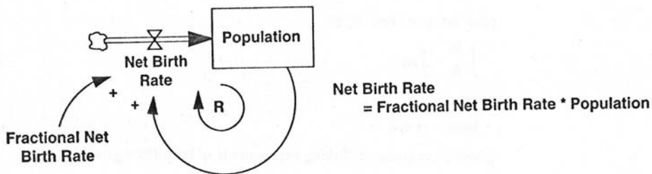
شکل (۸-۲): مثالهایی از ساختار سیستم‌های بازخوردی مثبت خطی درجه اول
