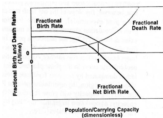
شکل (۸-۱۴): رابطه غیرخطی بین تراکم جمعیت و درصد نرخ رشد
