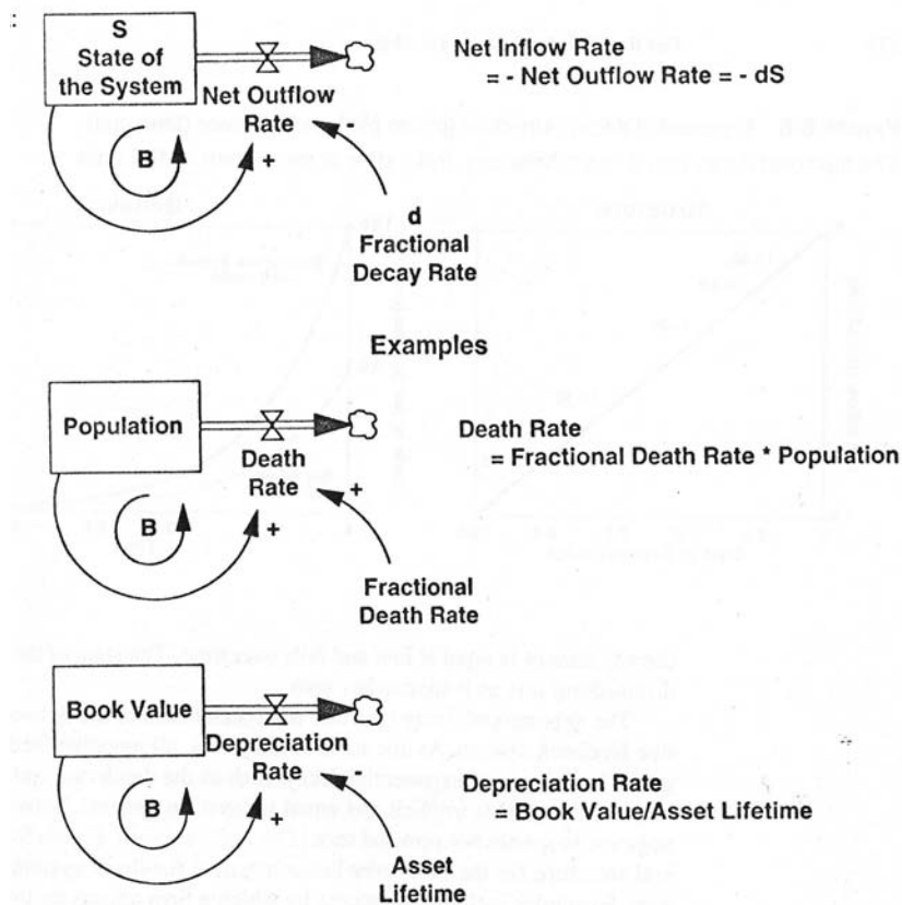
شکل (۸-۶): بازخورد منفی خطی درجه یک: ساختار و مثالها
